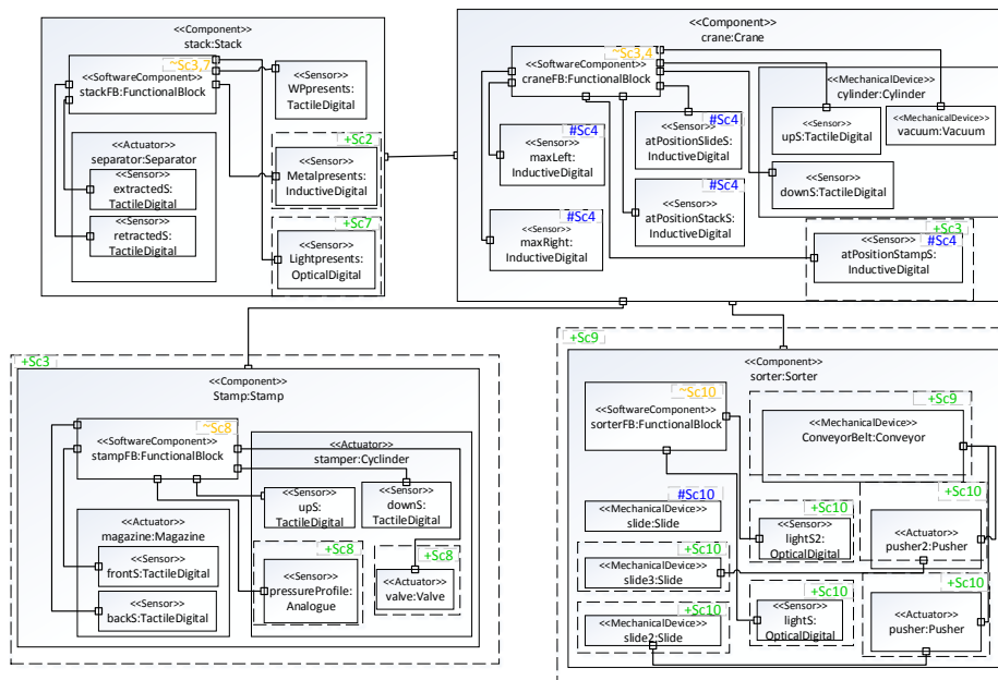
(a) SA model of the PPU
